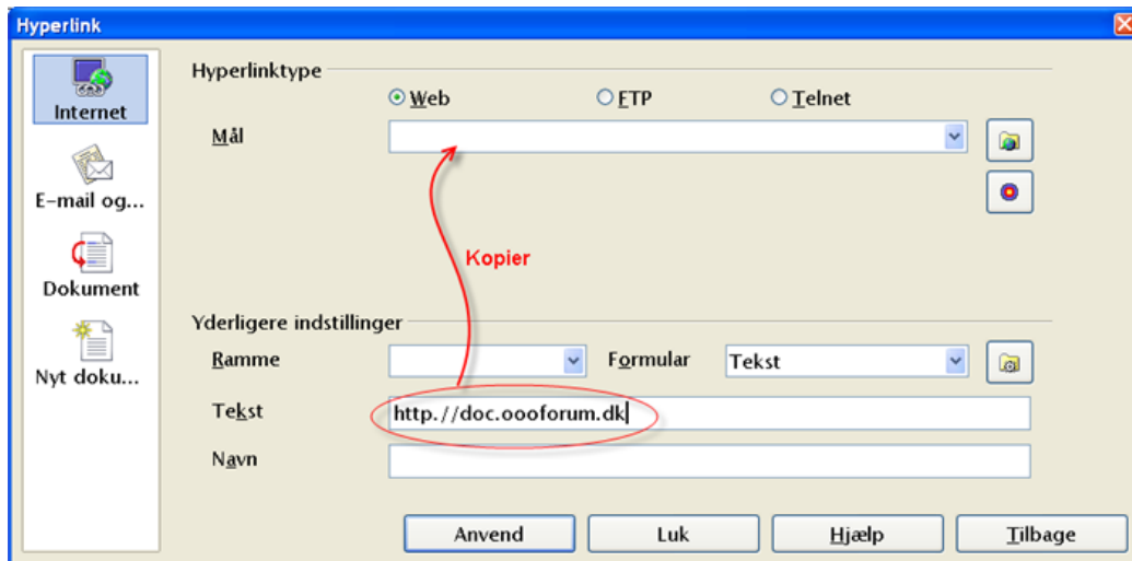
Figur 2. Dialogen hyperlink
