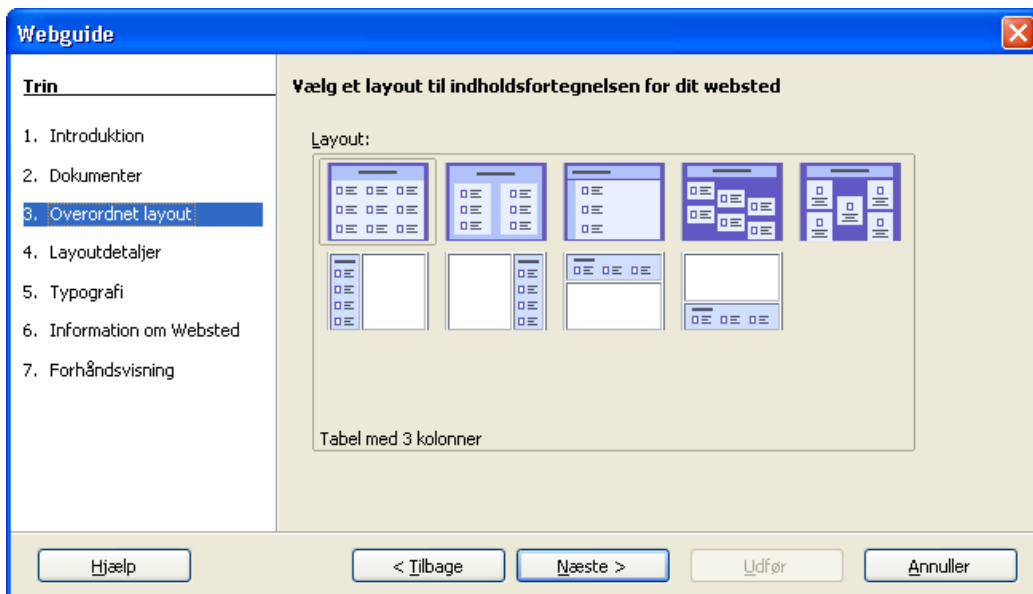
Figur 6. Webguide trin 3
